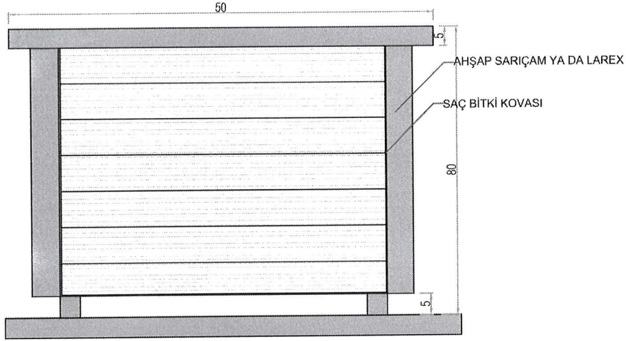
KESİT
